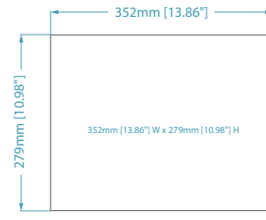
Cutout Dimensions
