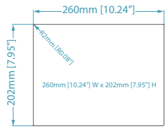
Cutout Dimensions
