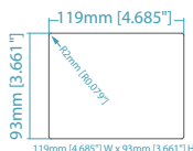
Cutout Dimensions
