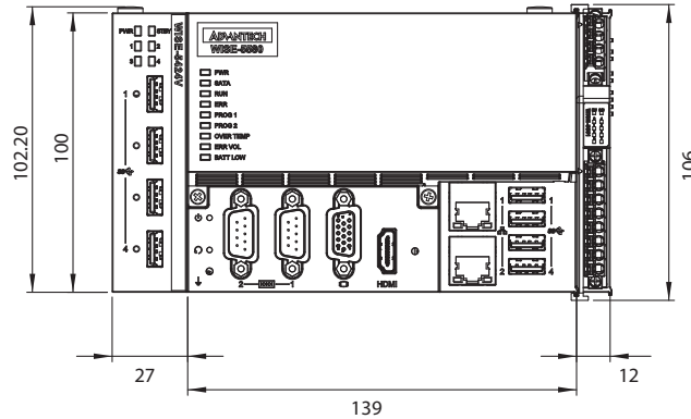
WISE-5580 CPU Module
