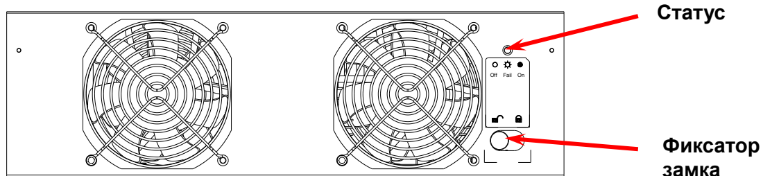
Рис.3-7 Силовой модуль. Вид спереди
