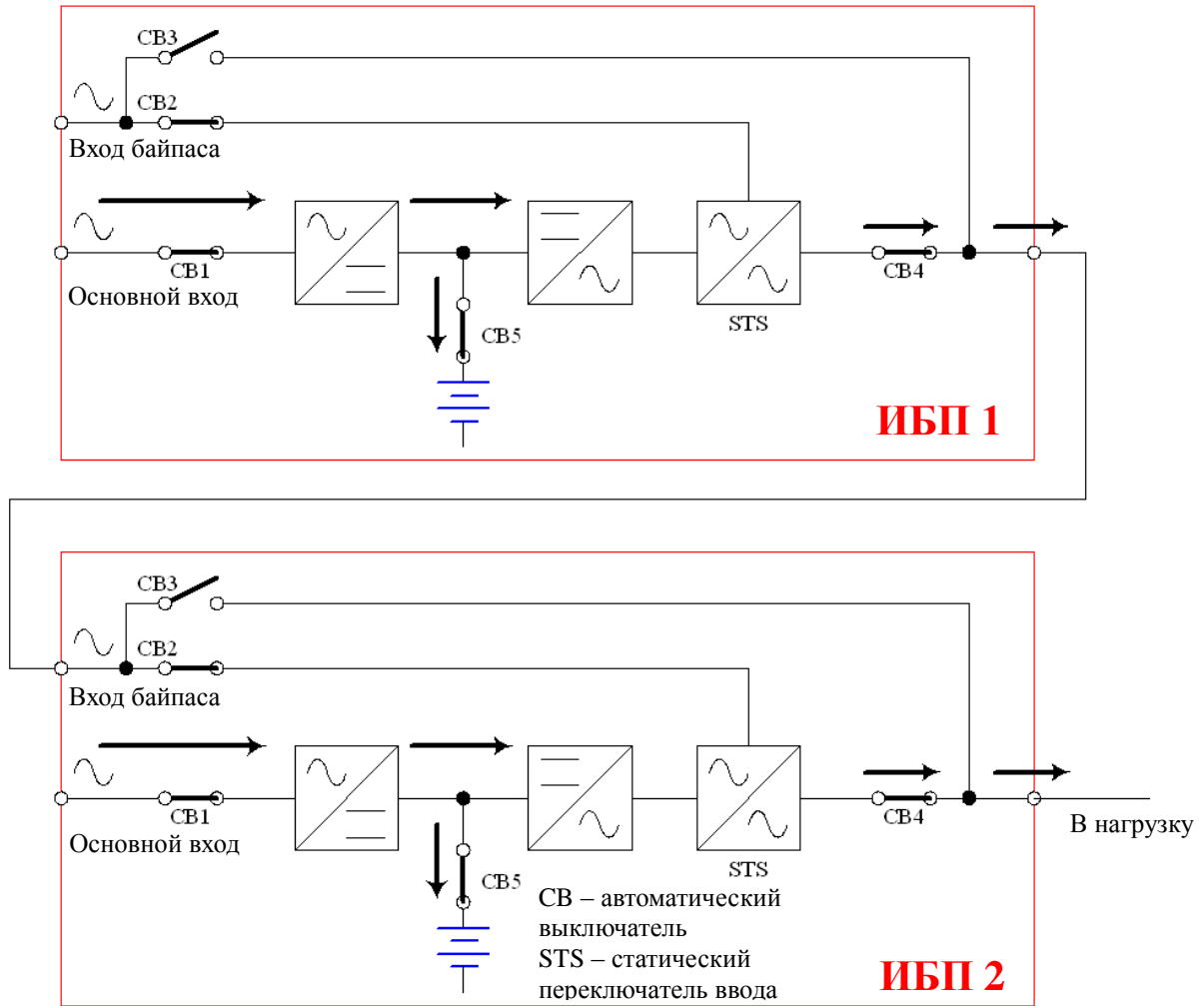
Рис.2-9 Система резервирования с несколькими последовательно включенными ИБП
