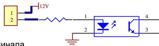
Рис.3-11 Схема REPO
