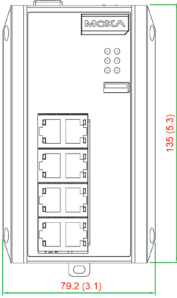
EDS-G508E
